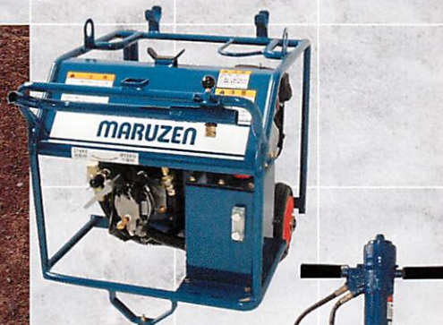
油圧パワーユニット U-070-1
