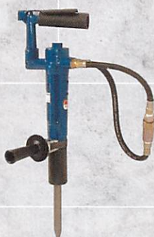
油圧ハンドブローカ BH-05B
